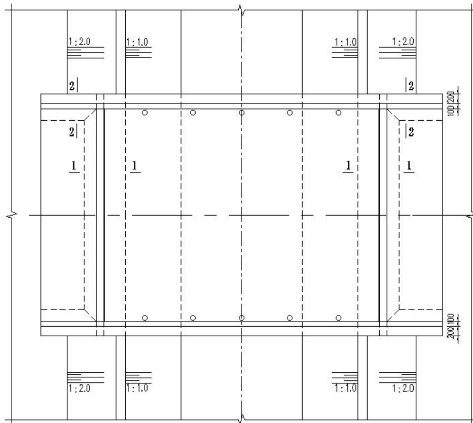
平面图 0 0.5 1.0 2.0m
