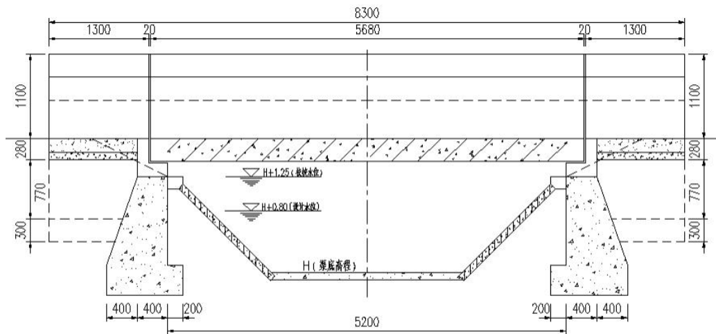
纵剖视图 0 0.5 1.0 2.0m
