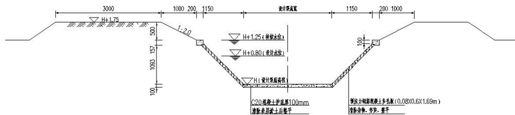
图 2-3 渠道护砌标准断面图
