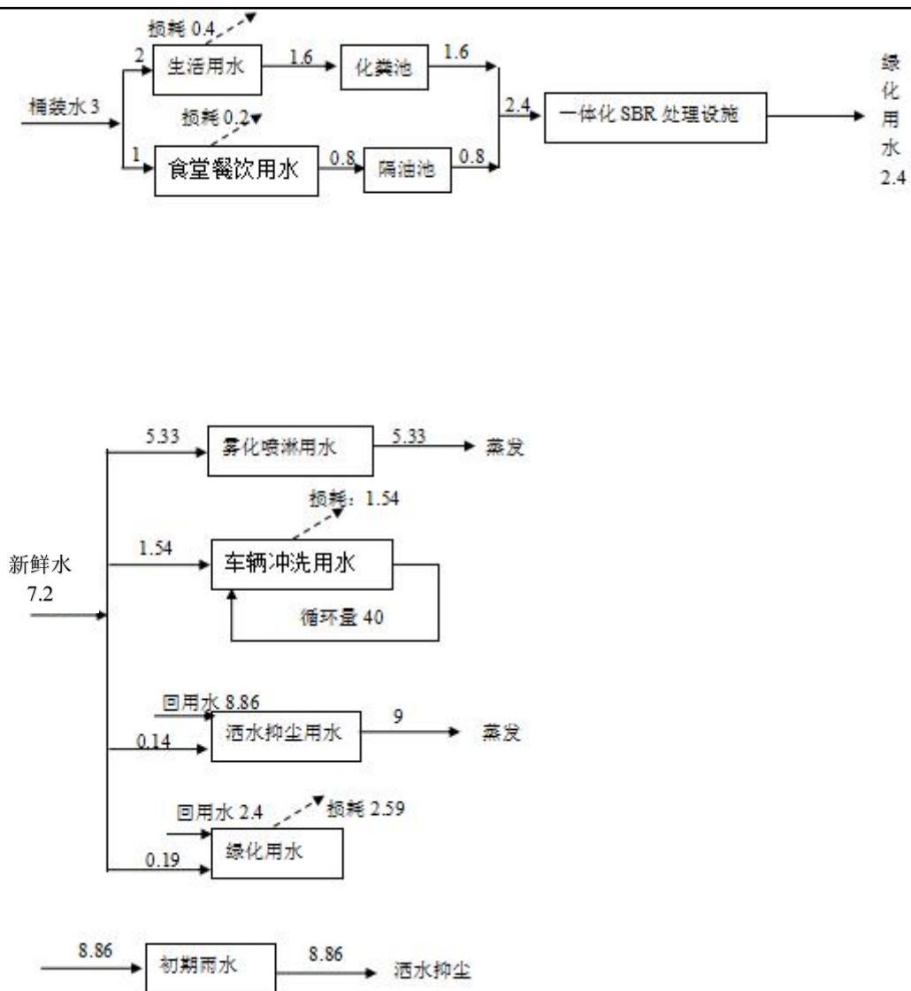
图 2-1 现有工程水平衡图（单位：t/d）
