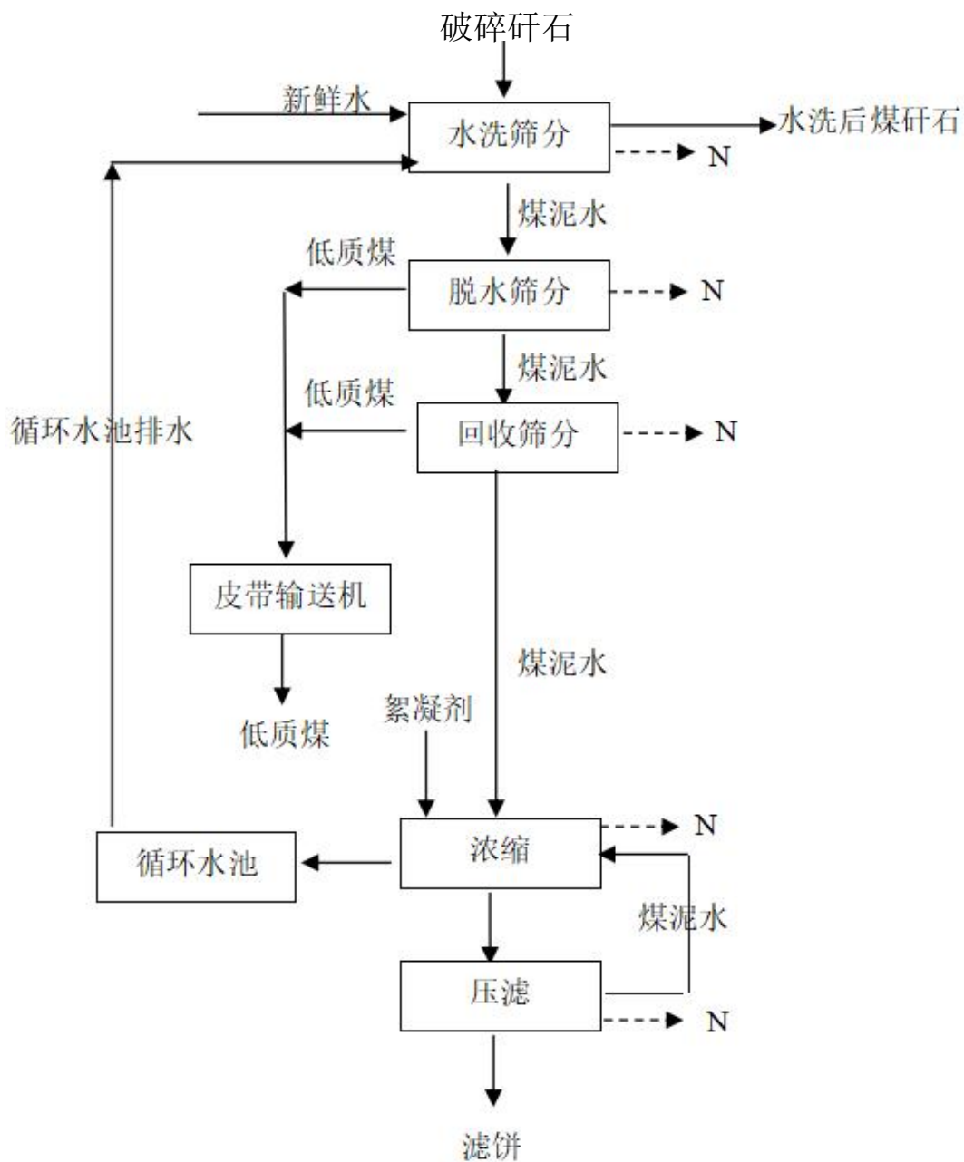
图 2-4 矸石洗选生产工艺流程及产污节点图
