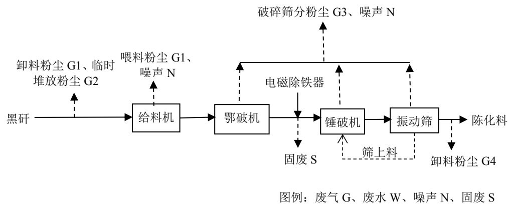
图 2-6 现有工程黑矸陈化料生产工艺流程及产污节点图 工艺流程简述
