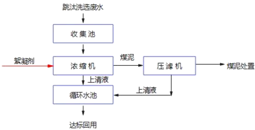
图 4-1 浓缩机污水处理工艺
