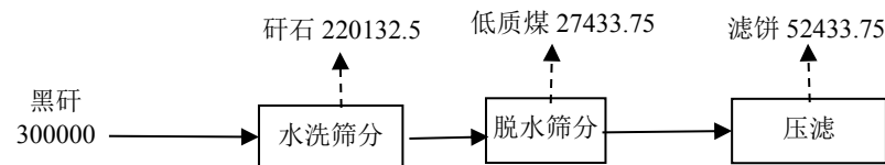
图 2-5 黑矸洗选生产物料平衡图 (t/a)
