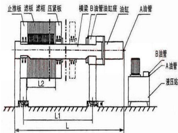
图 4-2 压滤机工作示意图
