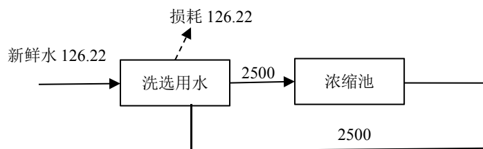
图 2-2 本项目水平衡图 （单位：t/d）
