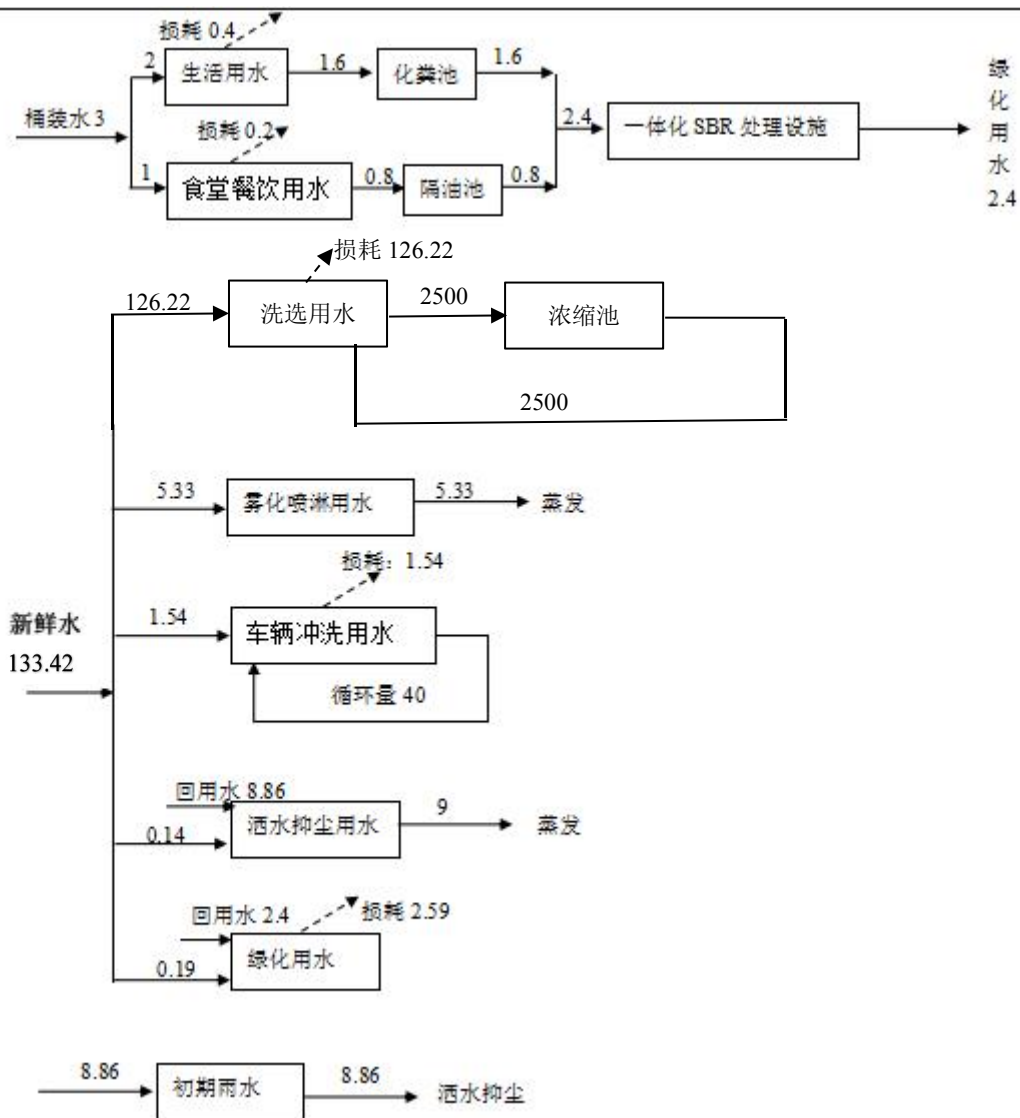
图 2-3 改建完成后全厂水平衡图 单位：t/d
